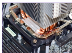
SUPOORTE FIXADO EM PLACA-MÃE
