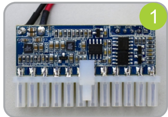
CN24. Conector 24P padrão ATX
