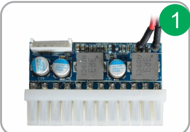
CN24. Conector 24P padrão ATX
