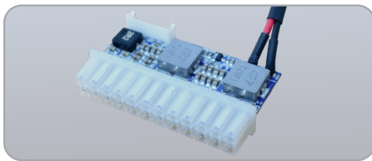
Placa conversora DC ATX Entrada 12V DC Saídas DC 5V, 12V, 3,3V, 5VSB e -12V
