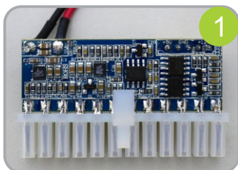
CN24. Conector 24P padrão ATX
