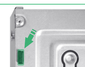
Trava para leitor de DVD
