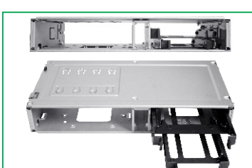
Vista do suporte das Baías tool less de 5.25" | 2.5" | 3.5"
