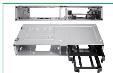
Vista do suporte das Baías tool less de 5.25" | 2.5" | 3.5"
