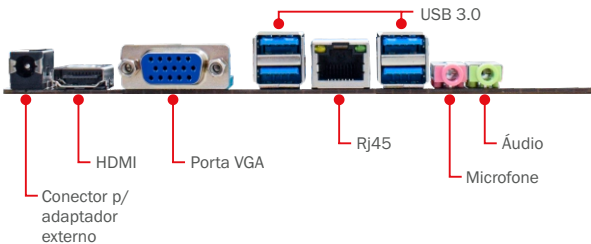
Conectores da placa-mãe
