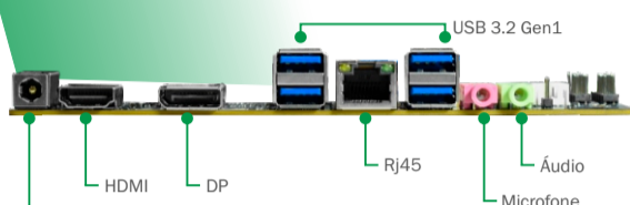
CONECTORES DA PLACA-MÃE
