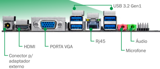
CONECTORES DA PLACA-MÃE
