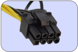
1 de 8 pinos PCI-E
