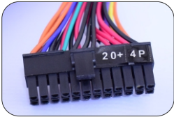
1 de 24 pinos (24p)
